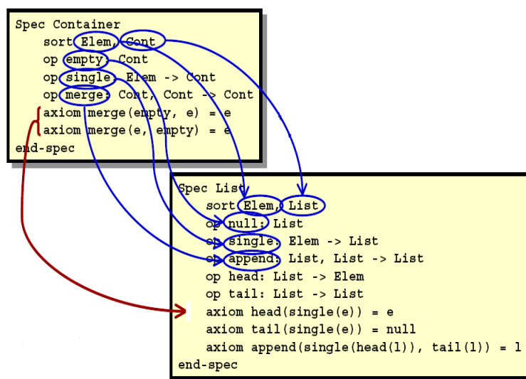
Рис. 2.1. Імплементація специфікацій морфізмів
